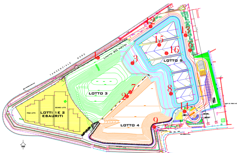
Fig. 18 - Punti di indagine relativi alle campagne di misura di COV e Composti organici solforati.
