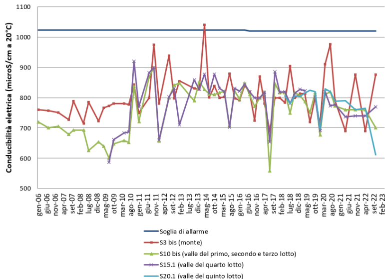
Fig. 11 - Valori di conducibilità elettrica della falda ( \mu\text{S}/\text{cm} a 20^\circ\text{C} ).
