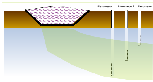
Fig. 10 - I piezometri sono in grado di monitorare la falda a differenti profondità.
