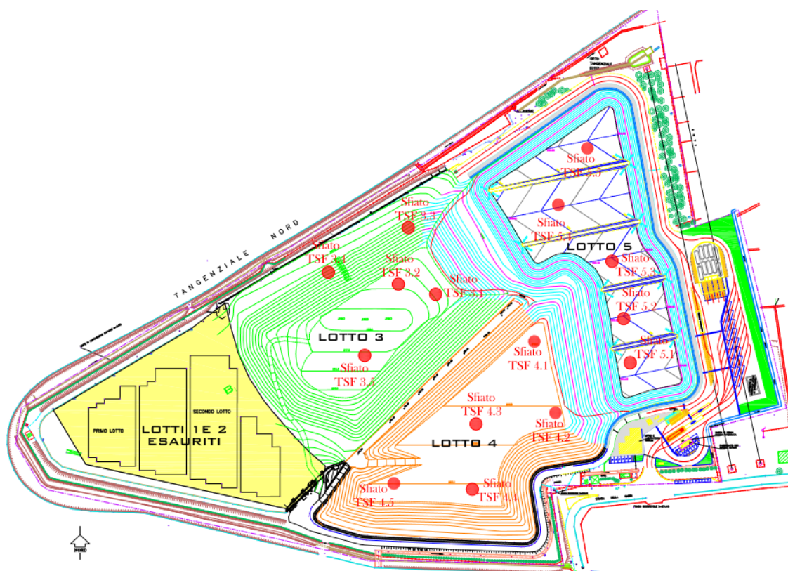
Fig. 17 - Planimetria sfiati - TSF
