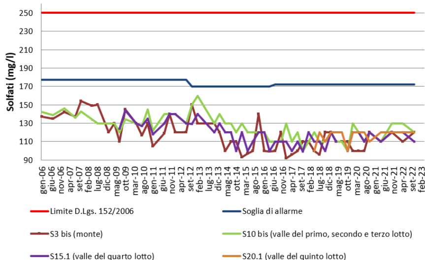
Fig. 12 - Concentrazione dei solfati in falda (mg/l).
