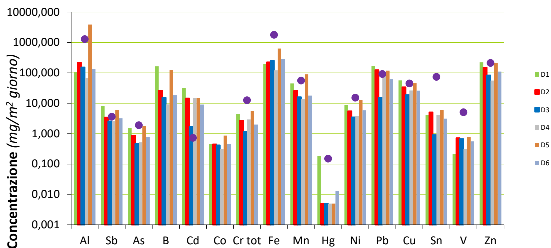
Fig. 21 - Comparazione dei valori rilevati nelle 5 campagne con i valori di bianco ( \mu\text{g}/\text{m}^2 \cdot \text{giorno} ).
