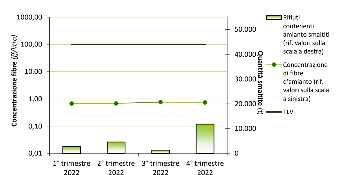
Fig. 22 – Monitoraggi ambientali confrontati con i rifiuti smaltiti e il TLV.
