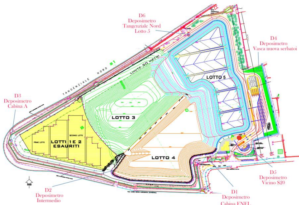
Fig. 20 - Ubicazioni dei deposimetri.
